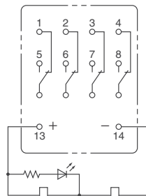
MY4(Z)N1/MY4(Z)IN1 (только модели для пост. тока)
