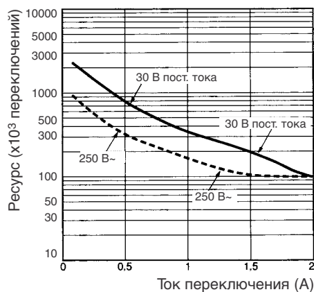
MY4 (индуктивные нагрузки)
