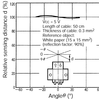
EE-SPY312/412
