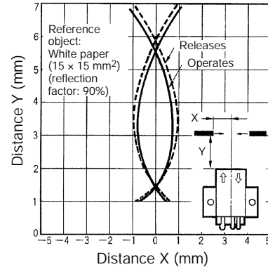
EE-SPY312/412
