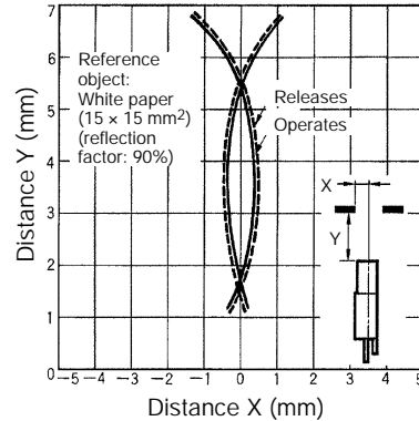
EE-SPY312/412
